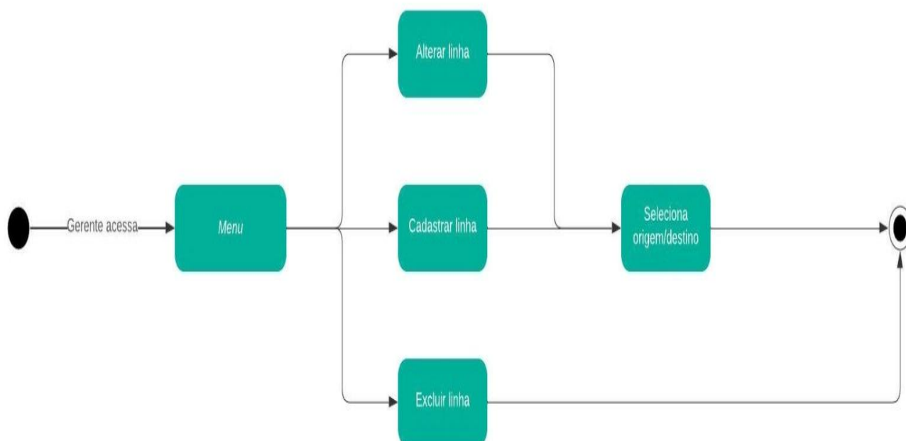
Figura 7: Diagrama de Atividades (Linha)
