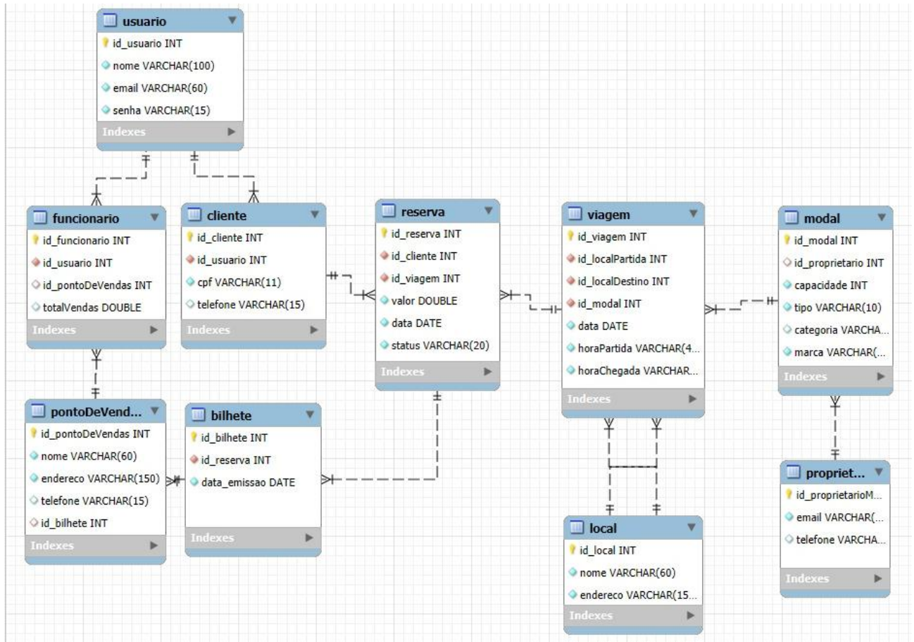
Figura 11 – Modelo Físico do Banco de Dados
