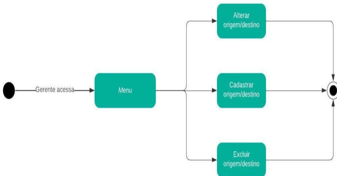
Figura 6: Diagrama de Atividades (Origem/Destino)
