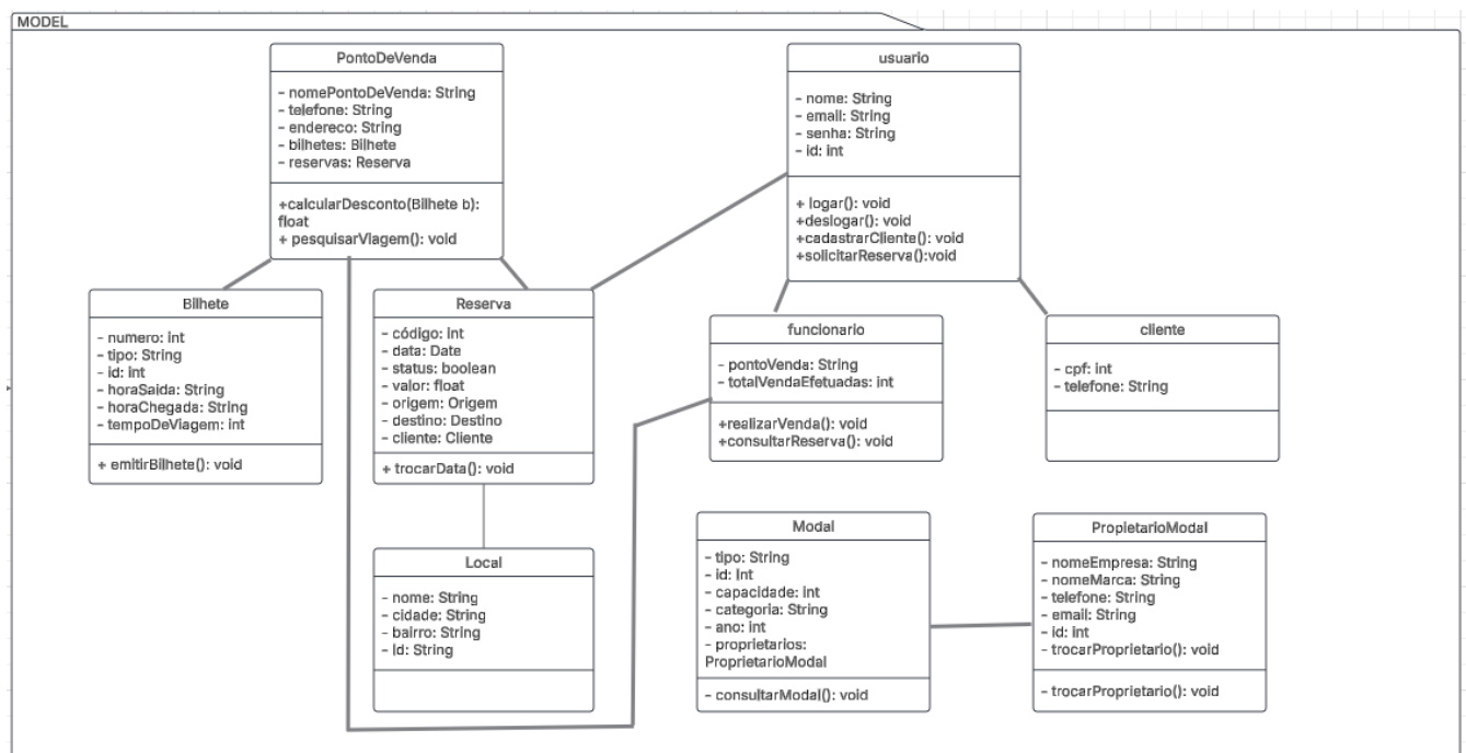
Figura 12- Diagrama de Classes padrão MVC
